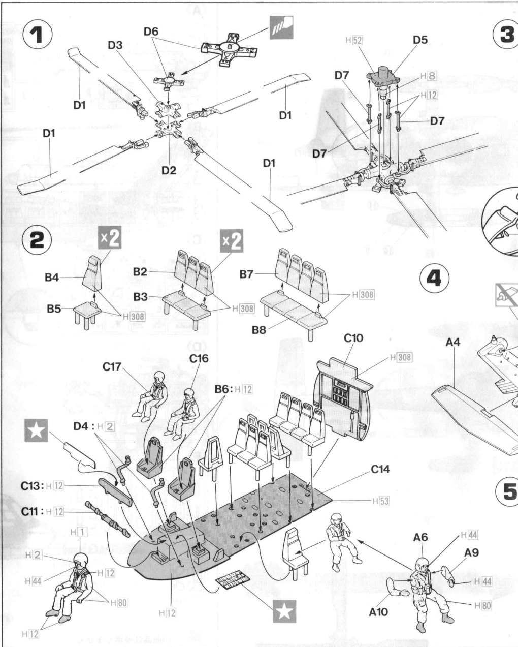
UH-60A BLACK HAWK
