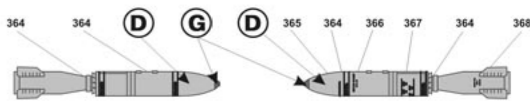
Бомба ФАБ-500ШР x 2 FAB-500ShR bomb x 2
