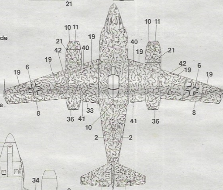
Messerschmitt Me 262 A-1a/U3 der Nahaufklärungs- gruppe 6 (NAGr. 6), Burg/b. Magdeburg, März 1945
