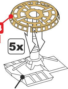
kit part F15.
