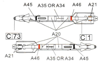
R-73空对空导弹 R-73 AA missile
