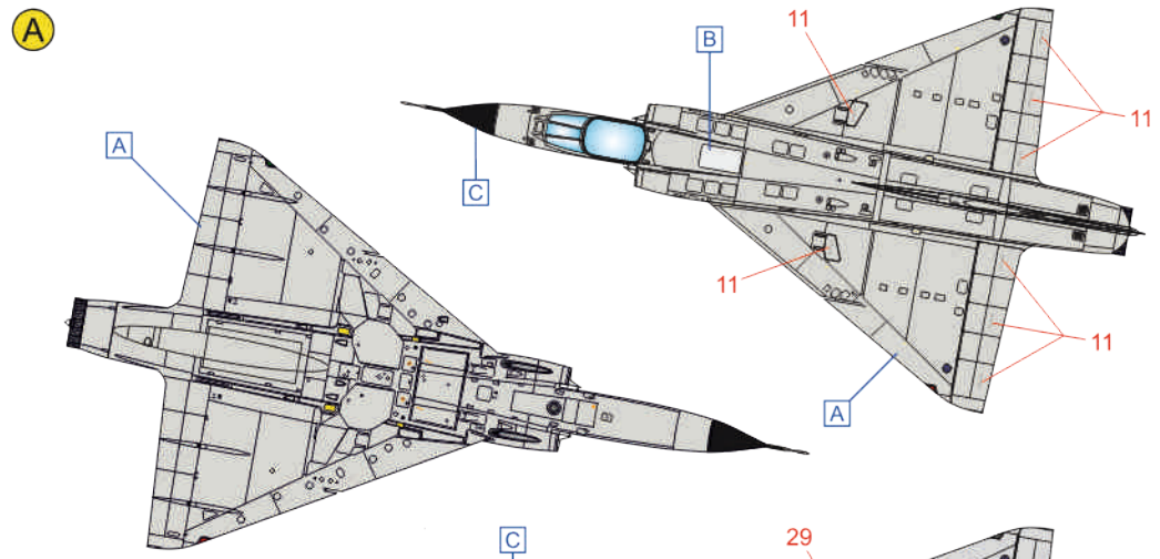
M Mirage IIIIEA, I-003, Argentinian Air Force, Grupo Aéreo 8 de Caza, Mariano Moreno AB, 1985
