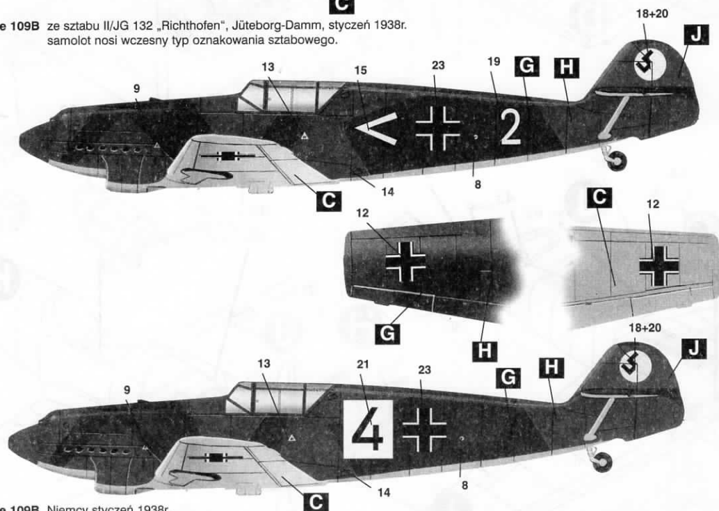
Me 109B Niemcy styczeń 1938r.
