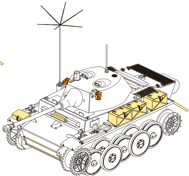
Luchs 5cm Vk1303
