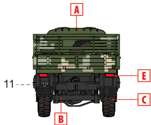
ЗіЛ-131, Збройні сили України, варіант камуфляжу з 2021 року ZiL-31, Armed Forces of Ukraine, camouflage version from 2021
