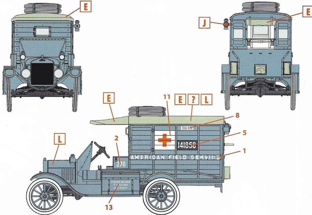
1. Модель Т 1917 г. санитарная (раннего выпуска), 30-й санитарный отряд, Франция, 1917 г. Model T 1917 Ambulance (early), SSU XXX, France, 1917
