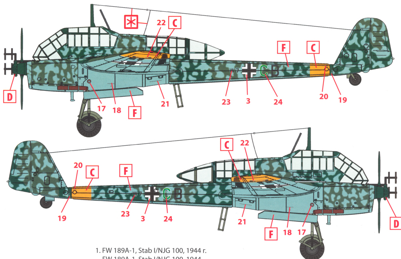
Стандартный камуфляж FW 189A-1 FW 189A-1 standard camouflage
