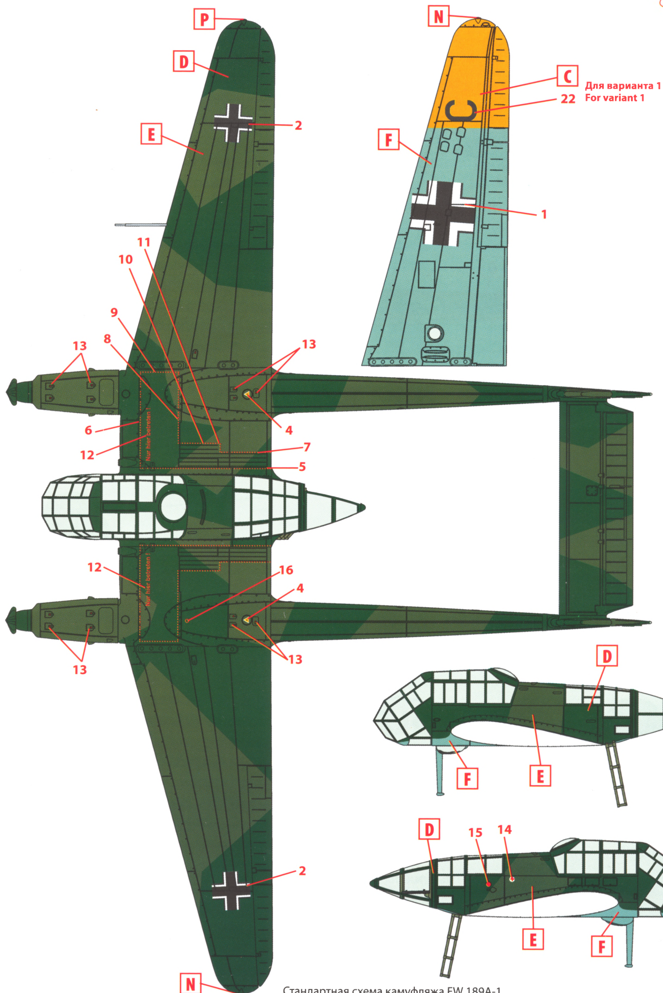
Стандартная схема камуфляжа FW 189A-1 FW 189A-1 standard camouflage scheme
