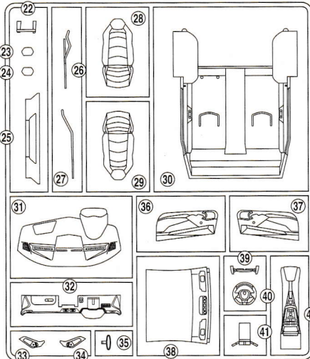
D部品 Tree D (12-1506-1)
