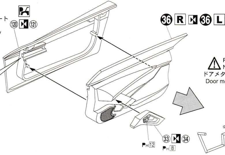
ドアサポートメタルステー Door suport metal stay
