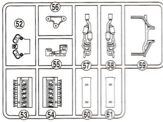
I部品 Tree I (12-1506-5)
