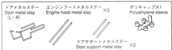
メタルステー小袋 Metal stay set
