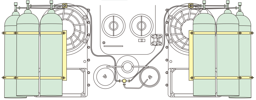
俯视图 Top view
