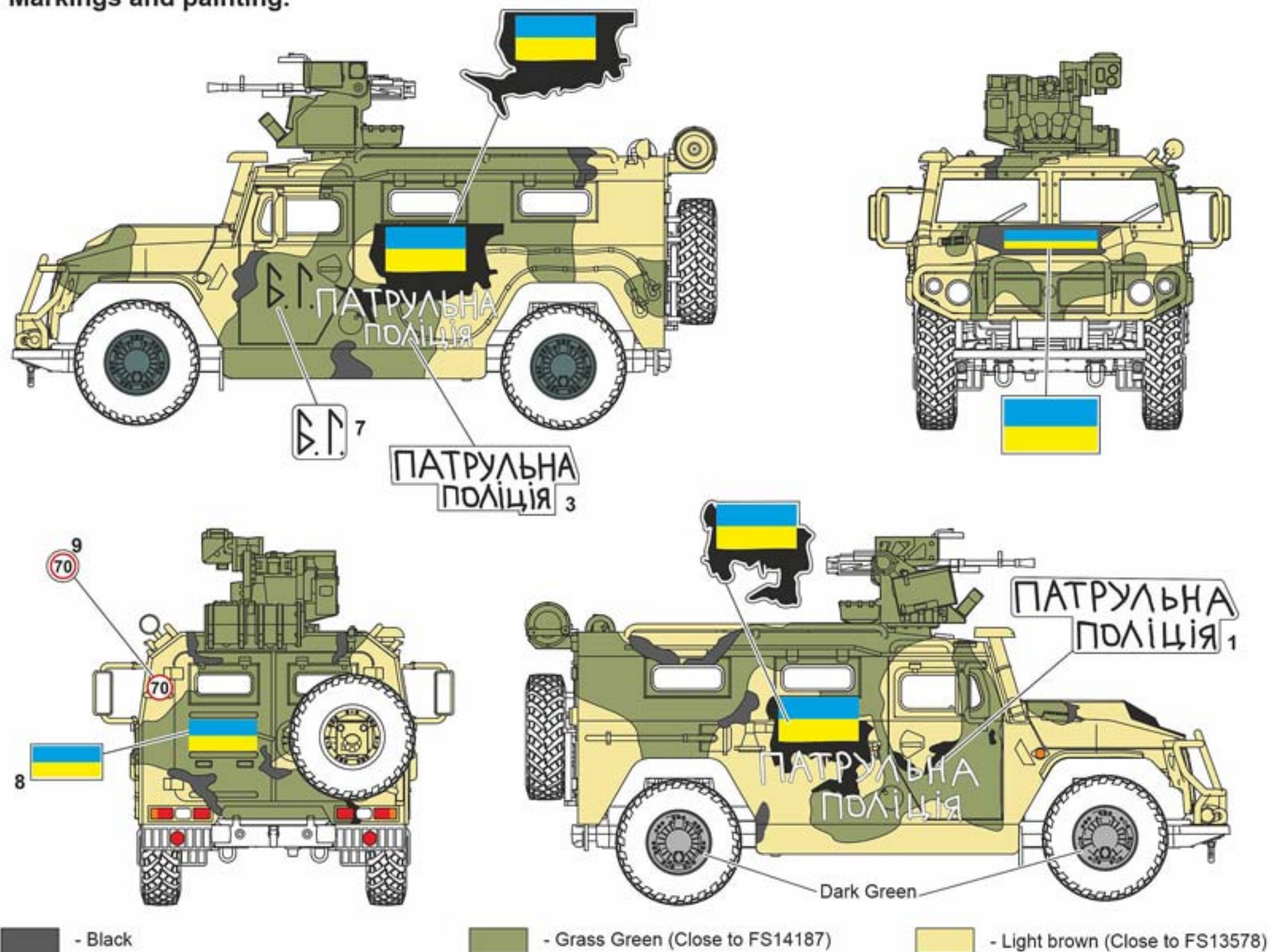
Tiger-M with heavy MG module Arbalet. Patrol Police. Mykolaiv Region. March 2022. Тигр-М з модулем Арбалет, Патрульна Поліція м.Миколаїв. Березень 2022.
