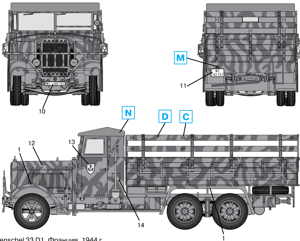
Henschel 33 D1, Франция, 1944 г. Henschel 33 D1, France, 1944
