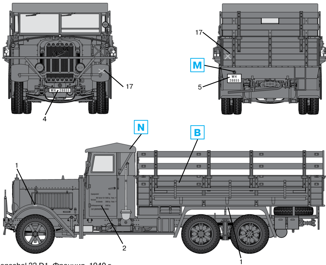
Henschel 33 D1, Франция, 1940 г. Henschel 33 D1, France, 1940
