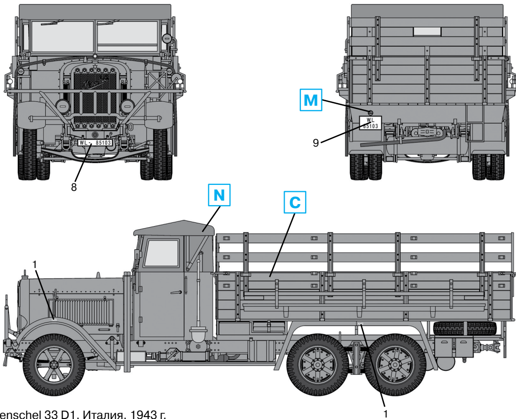
Henschel 33 D1, Италия, 1943 г. Henschel 33 D1, Italy, 1943
