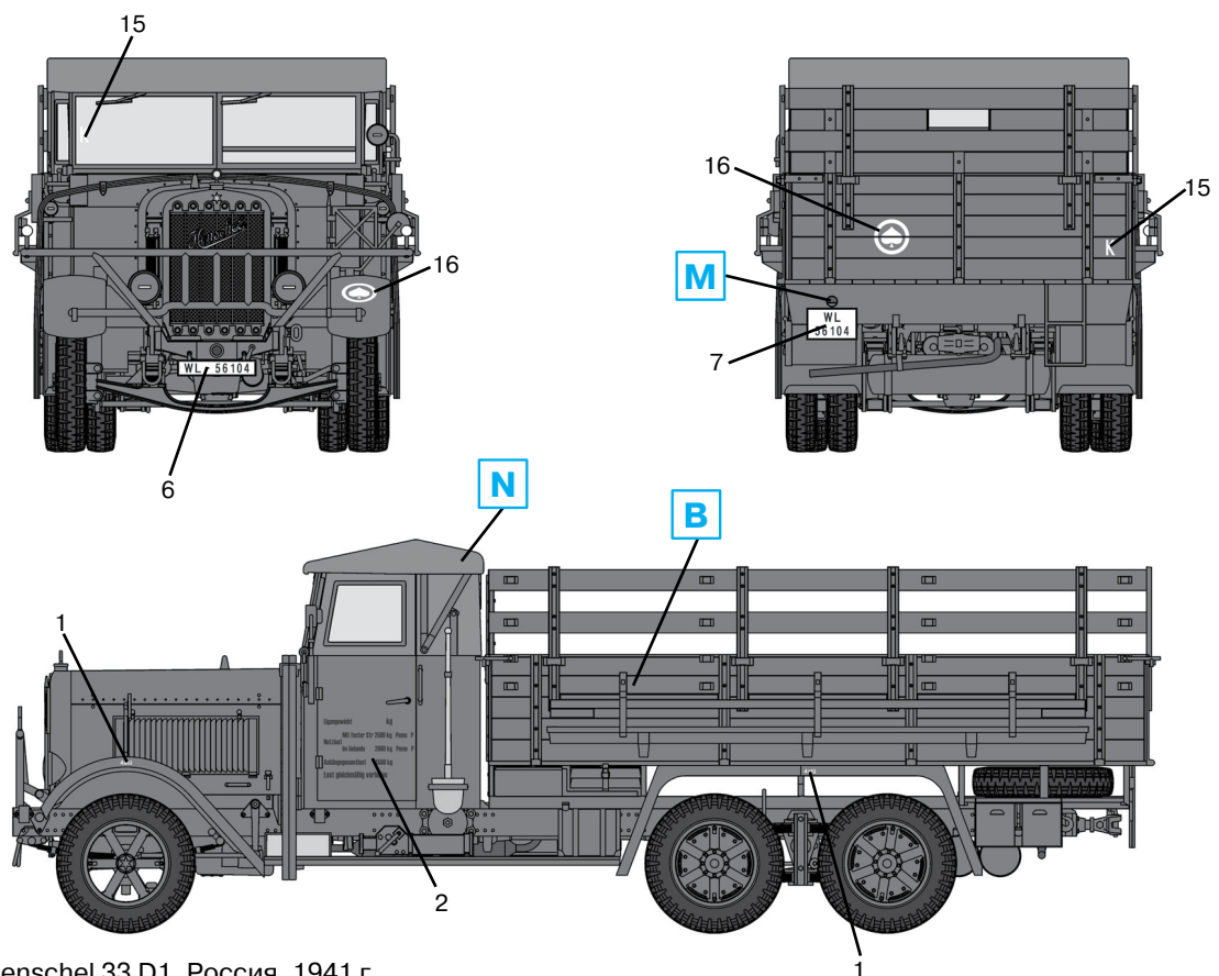
Henschel 33 D1, Россия, 1941 г. Henschel 33 D1, Russia, 1941
