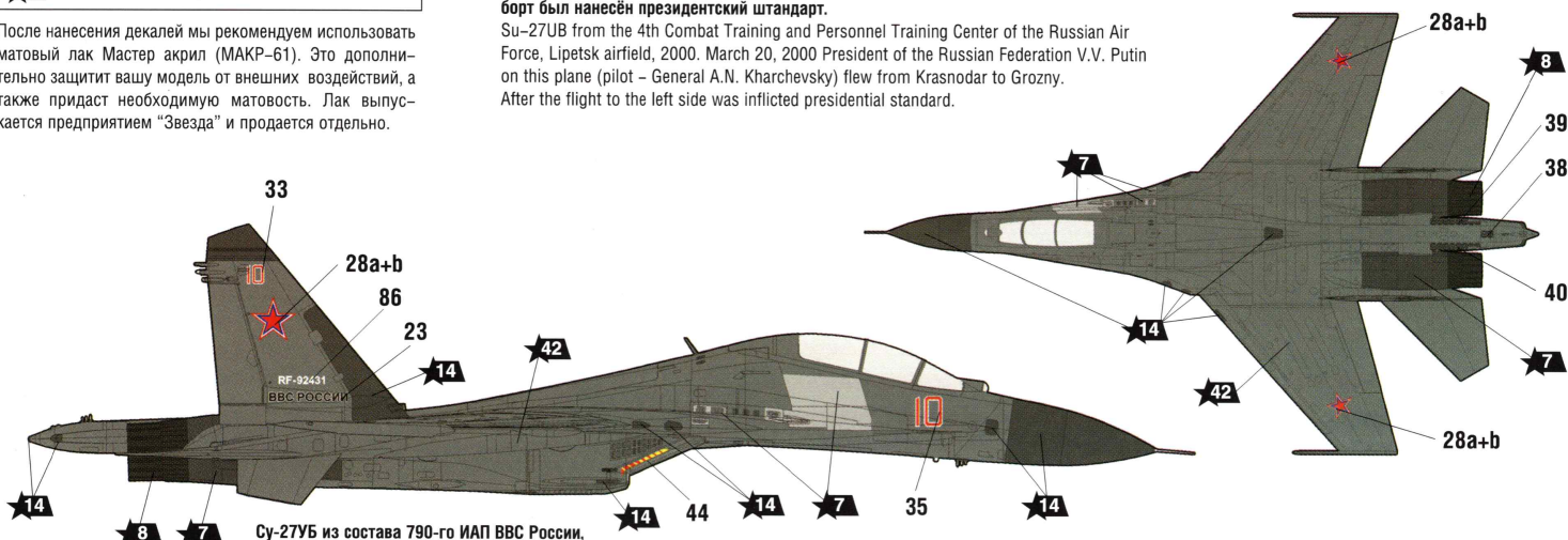
Су-27УБ из состава 790-го ИАП ВВС России, аэродром Хотилово, 2014 год.
