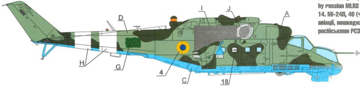
15. Mi-24P, Red 104, 11th Separate Army Aviation Brigade, Chernobaevka (Kherson), 2018 15. Mi-24П, червоний 104, 11 окрема бригада армійської авіації, Чернобаївка (Херсон), 2018 р.
