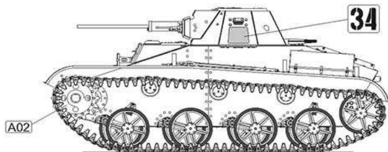
T-60 (zavod #37). Red Army. Central Russia. Summer 1942. Overall Soviet Khaki (4B0). T-60 (выпуск завода №37). РККА. Центральная Россия. Лето 1942г. 4Б0.
