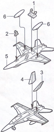
F/A-18E
