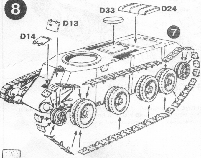
Схема сборки траков Circuit of tracks assembly
